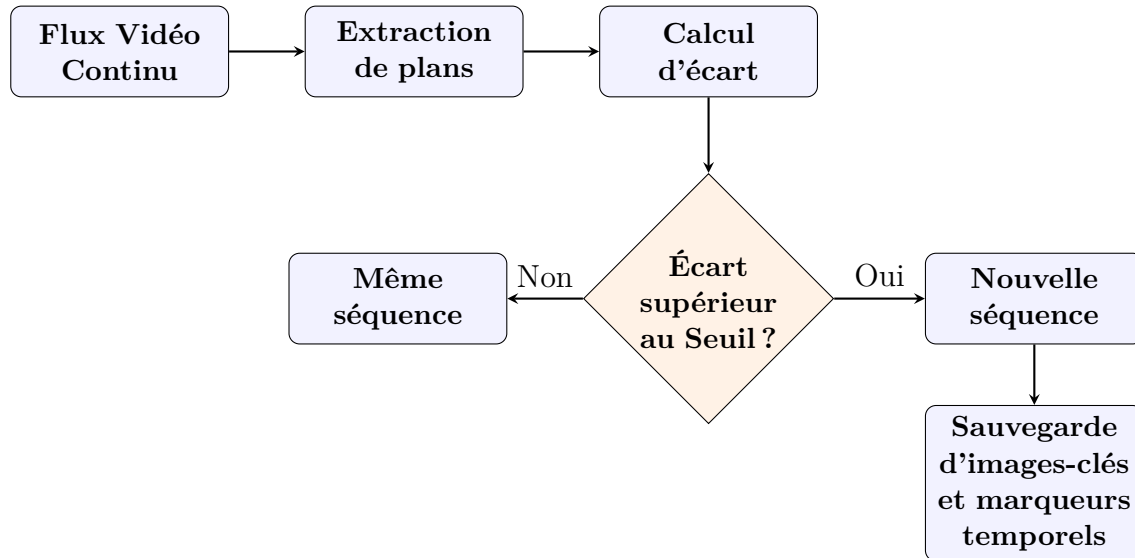
Figure 4.1 - Schéma du processus de détection de coupures et d'extraction d'images-clés par PySceneDetect
